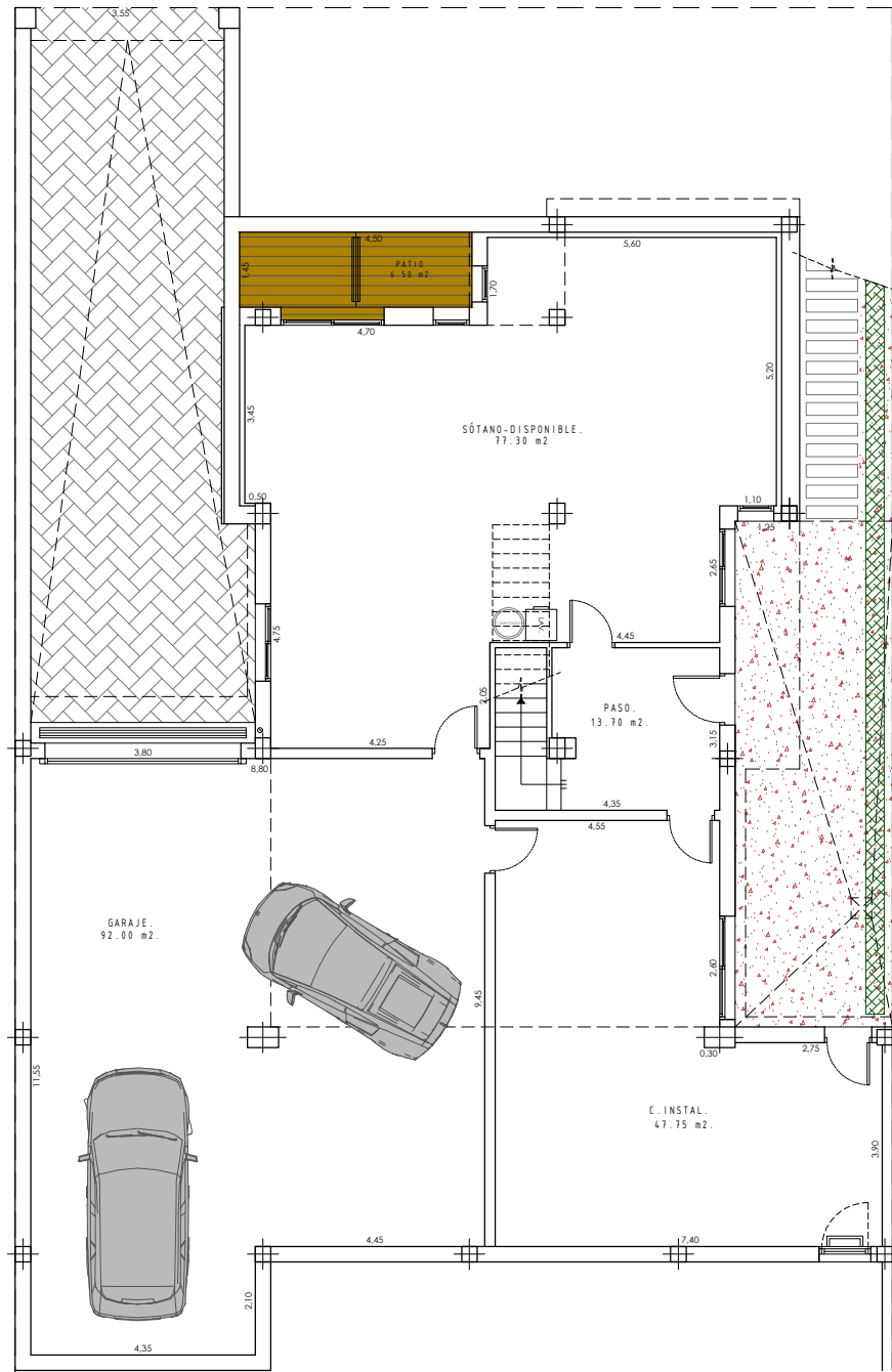
PLANTA SÓTANO
