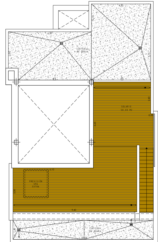
PLANTA CUBIERTA
