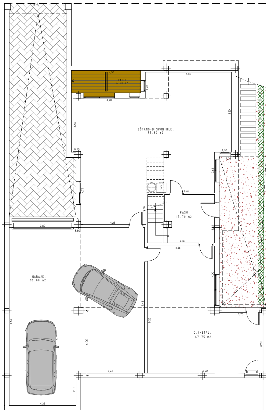
PLANTA SÓTANO
