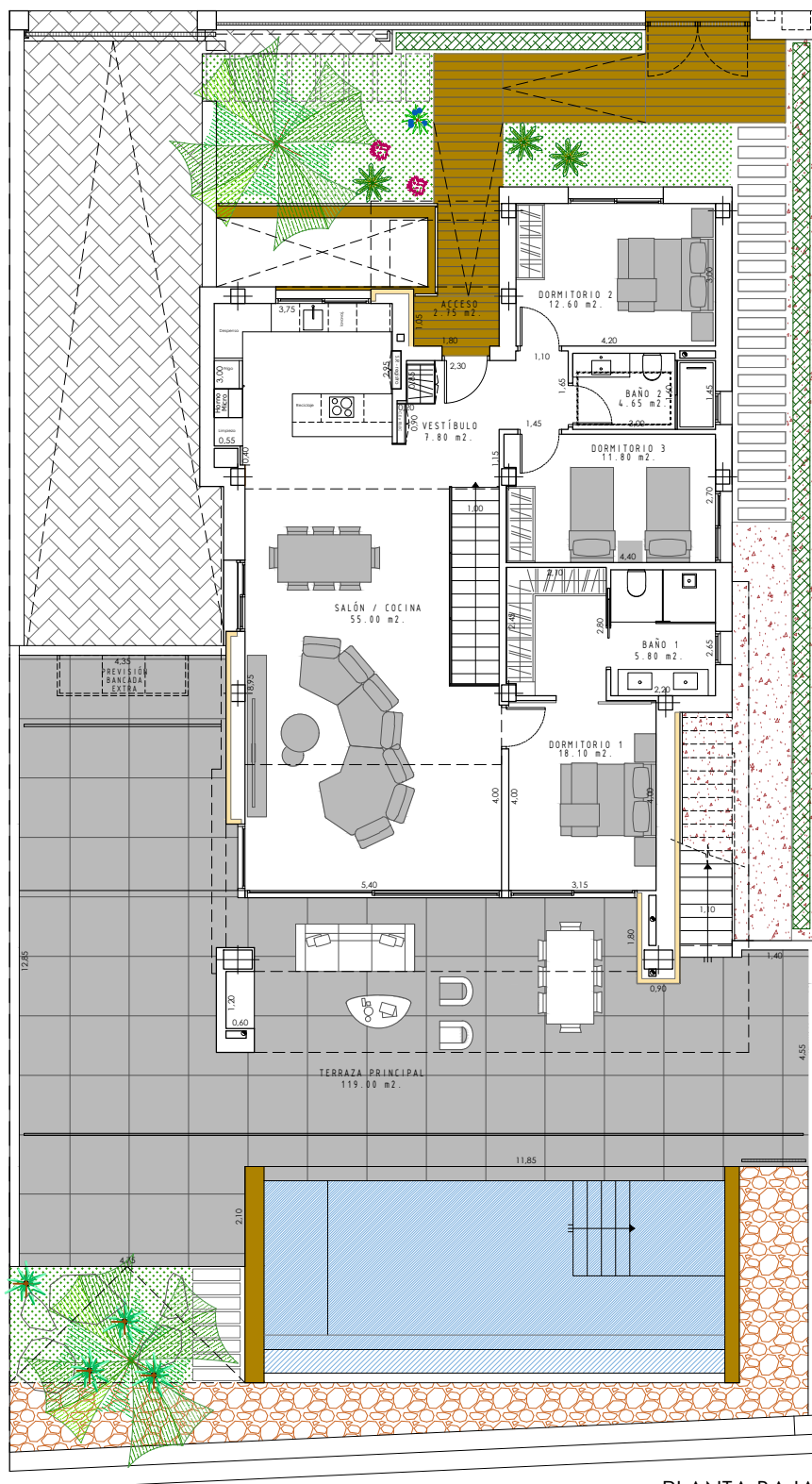
PLANTA BAJA
